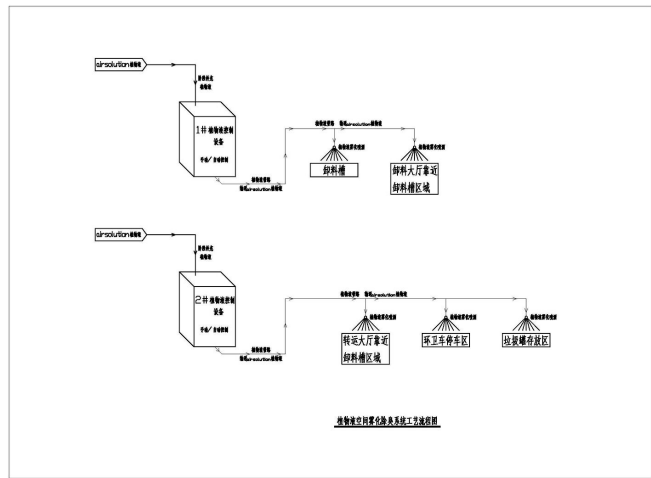
植物液空间雾化除臭系统工艺流程图
