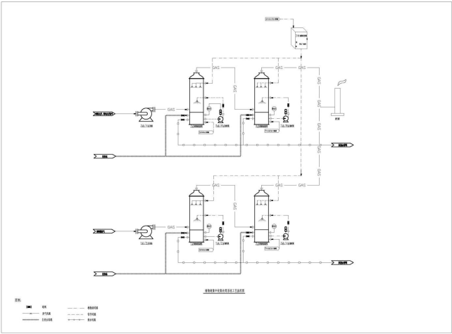
植物液集中收集处理系统工艺流程图
