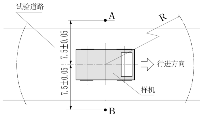
图3 噪声测量方法
